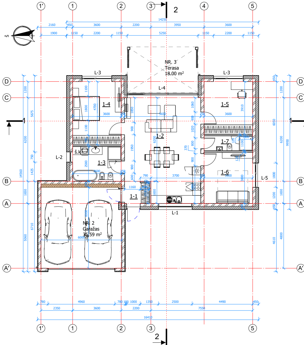
Pirmo aukšto planas M 1 : 100
