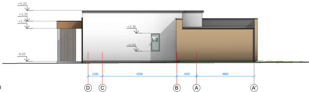
Fasadas D-A M 1 : 100
